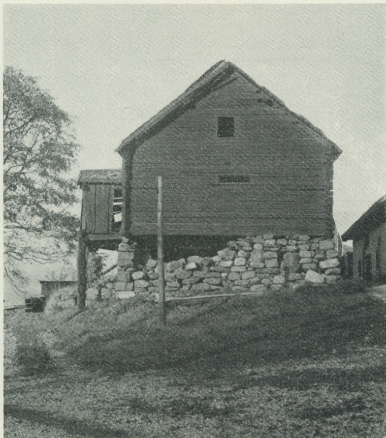
Trots förfallet är källarboden på Eka ett ståtligt byggnadsminnesmärke. En vindskada har fallit ned och den andra har lossnat och följer snart efter. Muren i gavelväggen håller på att rasa och av trapphuset är ej mycket kvar. Foto okt. 1959 Ingalill Granlund.
