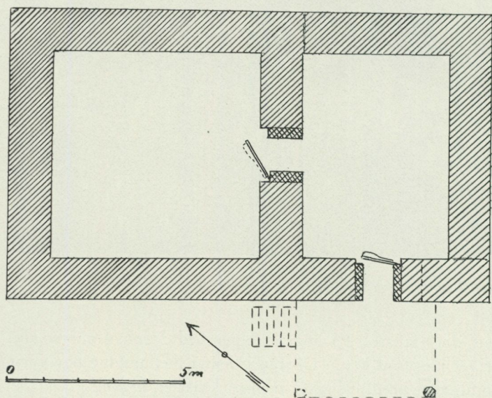
Plan av Ekaboden. Nedtill källaren, upptill våningen ovanför. Uppmätning 1957 och 1959 av Olle Homman.
