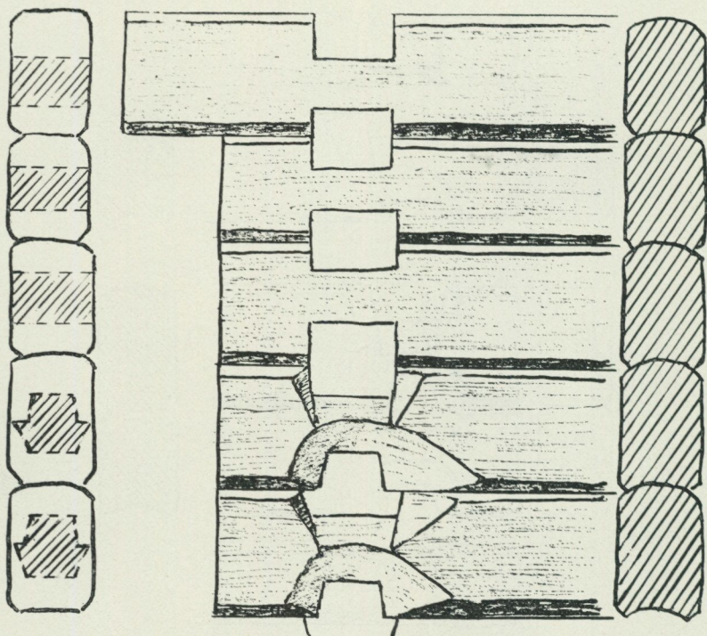
Detalj av knuten i bodens nordöstra hörn. De tre översta stockarna i norra långväggen har vertikal dubbelhaksknut utan betta och är ej vittrade. Teckning 1959 av Olle Homman.
