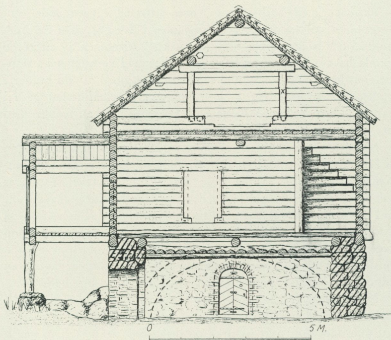
Sektion av källarboden på Eka. Vid x är året 1854 skrivet med rödkrita. Uppmätning 1957 och 1959 av Olle Homman.
