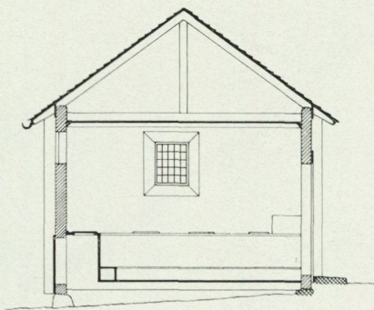
14—15. Ett avträde från 1700-talet för nio personer. Den kvadratiske grundplanen med bänkar utmed tre sidor för tankarna till ett konferensrum, Apertin, Värmland. Foto av interiören, se fig. 24. Uppmätning från 1960.
