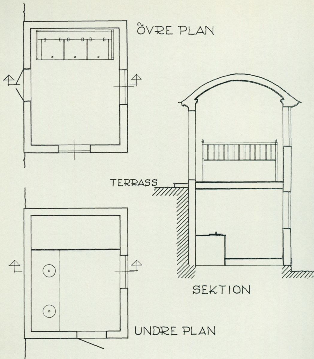
18. Uppmättningsritning av tvåvårigt avtråde på Vallstanäs herrgård i Norrsunda socken, Uppland. Övre planet med ingång från gårdsplanens terrass är avsett för herrskapet. Bänken är där utformad som en pinnsoffa. Undre planet nedanför terrassen är för tjänstefolket och något enklare inrett.
