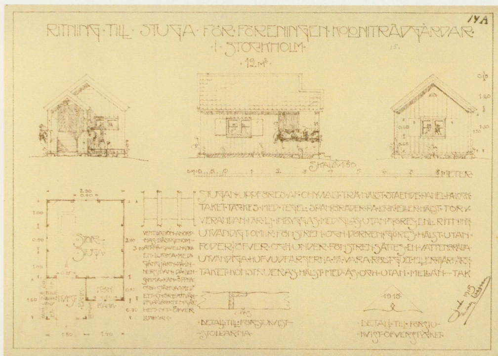
Ritning om 12 m 2 upprättad av Einar Larson 1915. Ritningen visar stugan från olika sidor samt i plan. Av texten framgår också i vilket material stugan skulle uppföras och i vilka färger den borde målas. Ritning från Gat- och fastighetskontoret i Stockholm.
